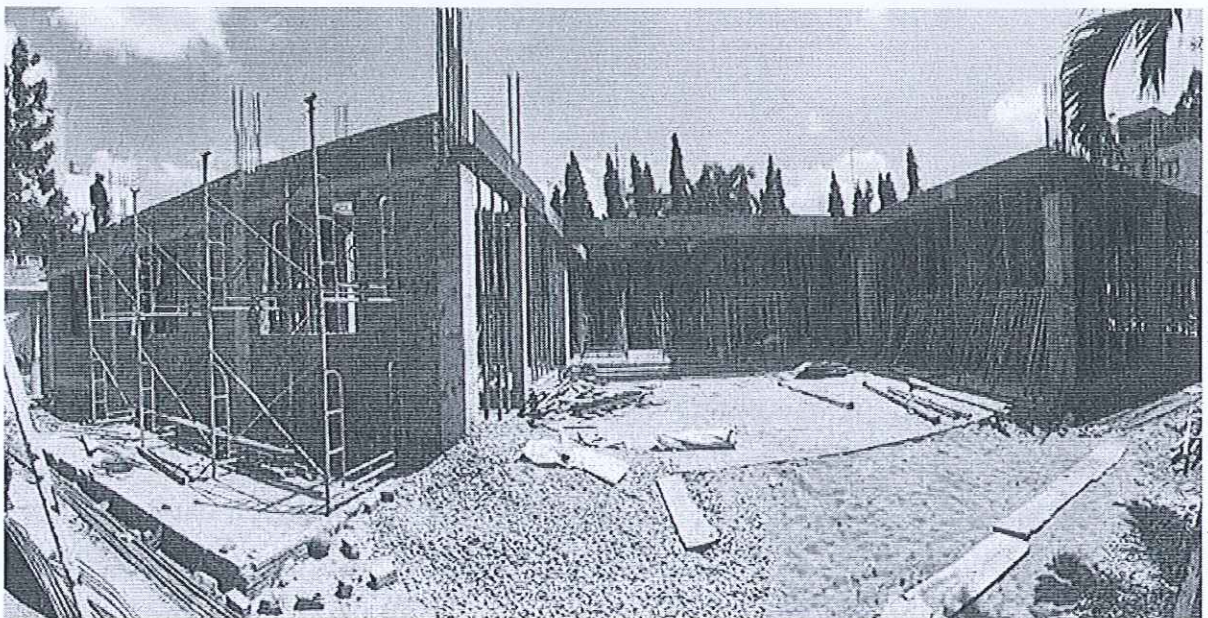
Thi công xây dựng mới Trường Mầm non 12, Quận 3
