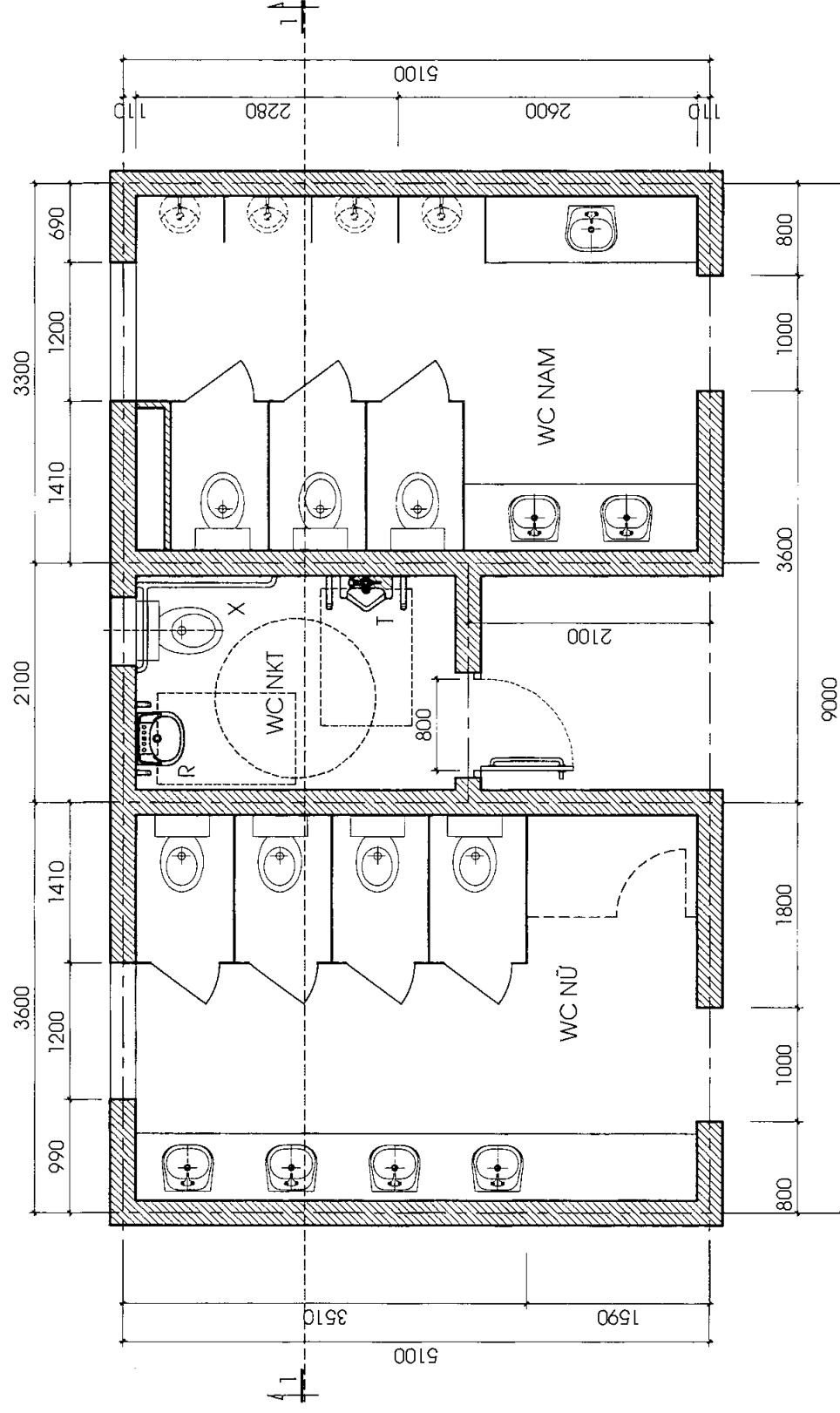
MẶT BẰNG
