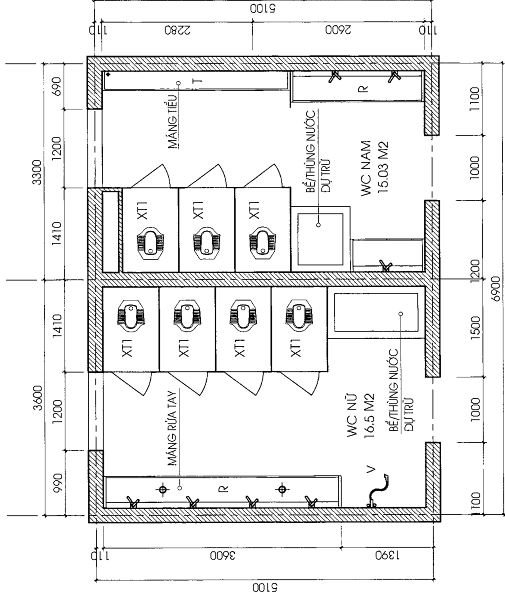
MẶT BẰNG 1/2
