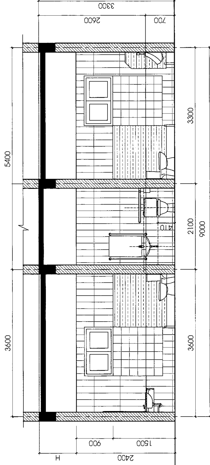
MẶT CẮT 1-1
